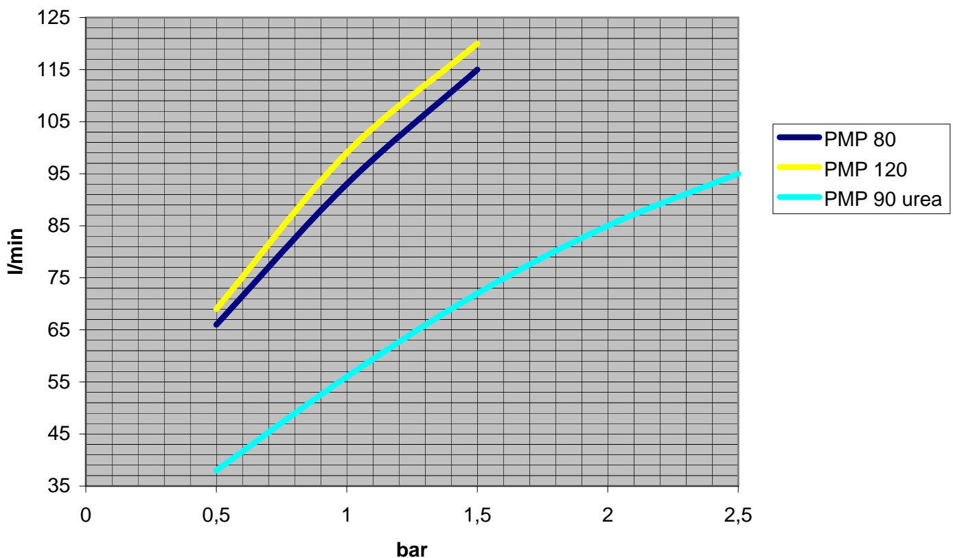
Diagramma pressione-portata
